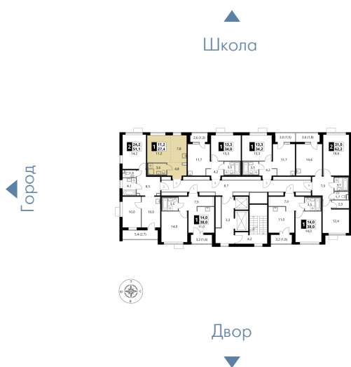
ПЛАНИРОВКА ЭТАЖА
